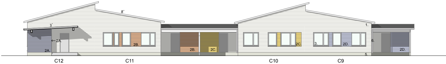
JULKISIVU KOILLISEEN
