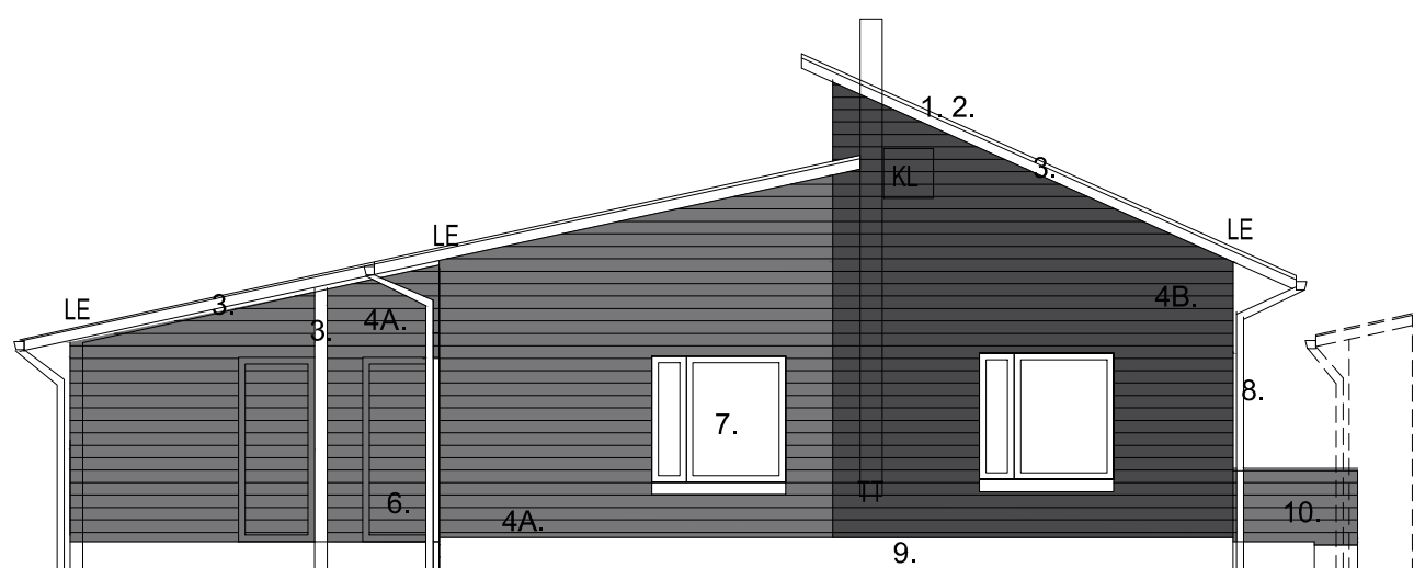
SISÄÄNKÄYNTIJULKISIVU ITÄÄN
