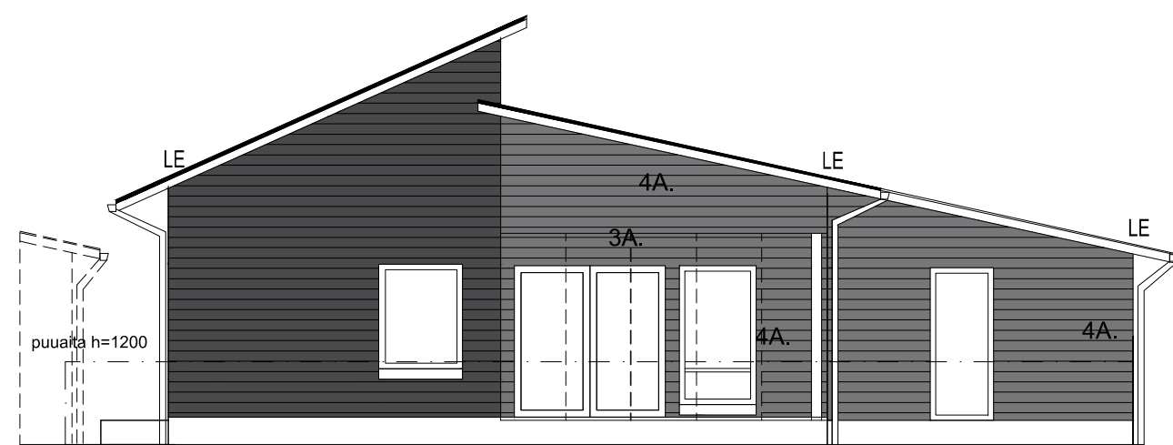
PIHAJULKISIVU LÄNTEEN
