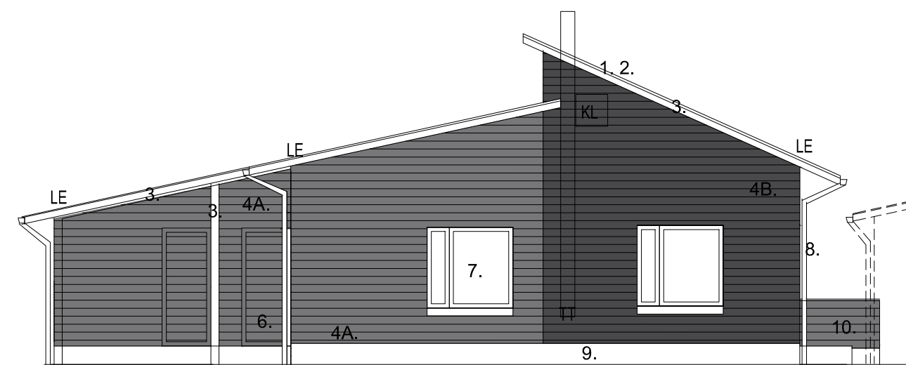
SISÄÄNKÄYNTIJULKISIVU ITÄÄN
