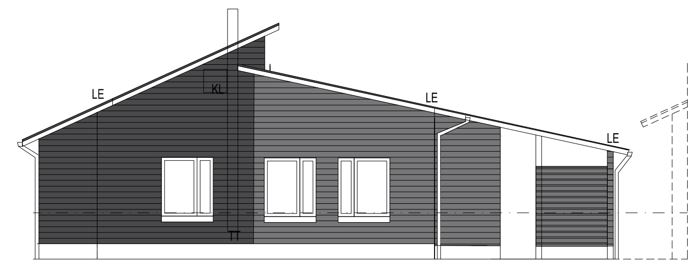
JULKISIVU KOILLISEEN
