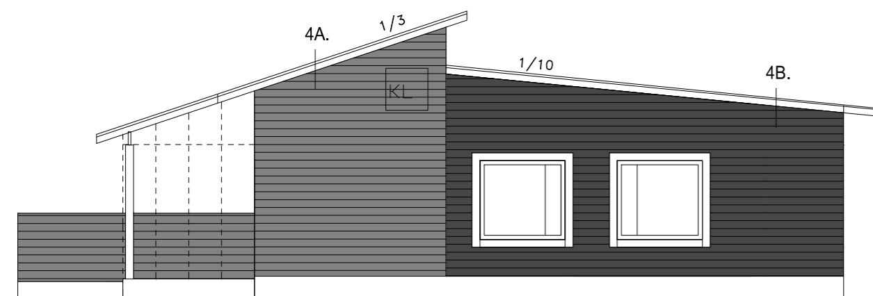
PÄÄTY ETELÄÄN
